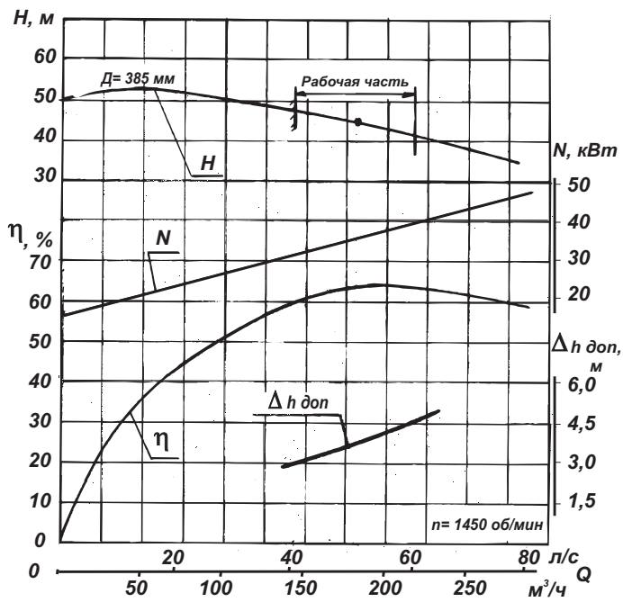
Характеристика насоса КСО 180-45
