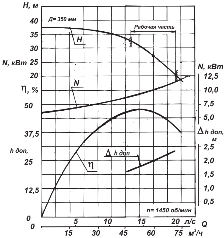
Характеристика насоса КСО 60-27
