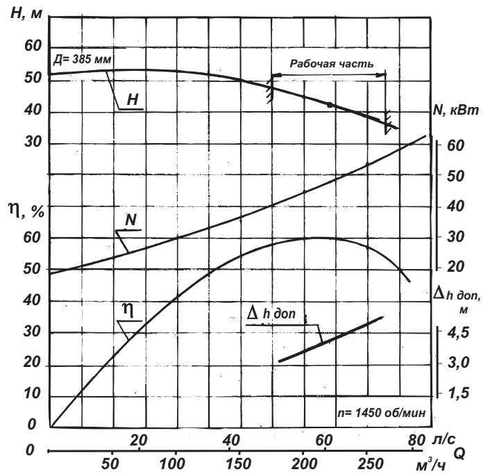
Характеристика насоса КСО 220-42
