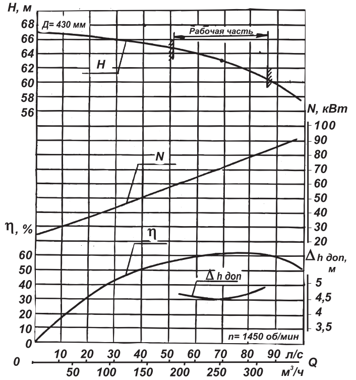
Характеристика насоса КФС 250-63
