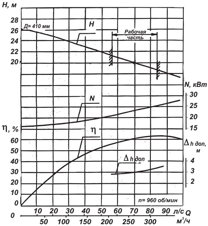
Характеристика насоса КФС 250-20
