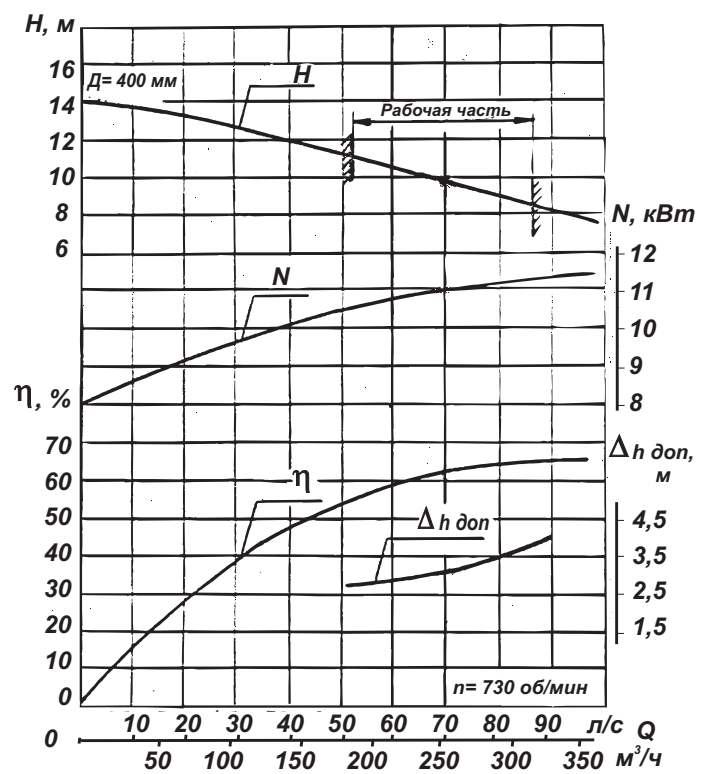
Характеристика насоса КФС 250-10
