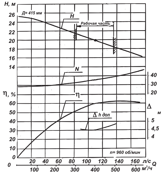
Характеристика насоса КФС 400-20
