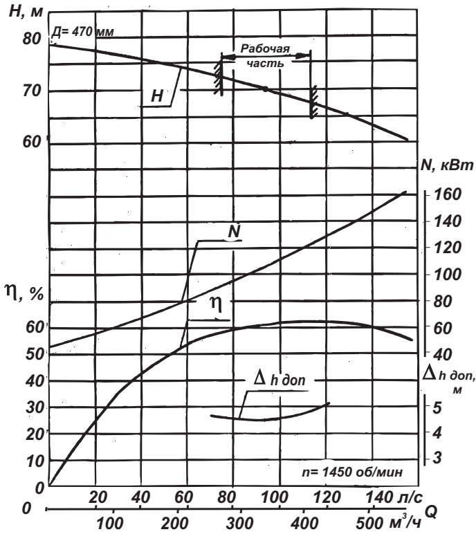
Характеристика насоса КФС 340-70
